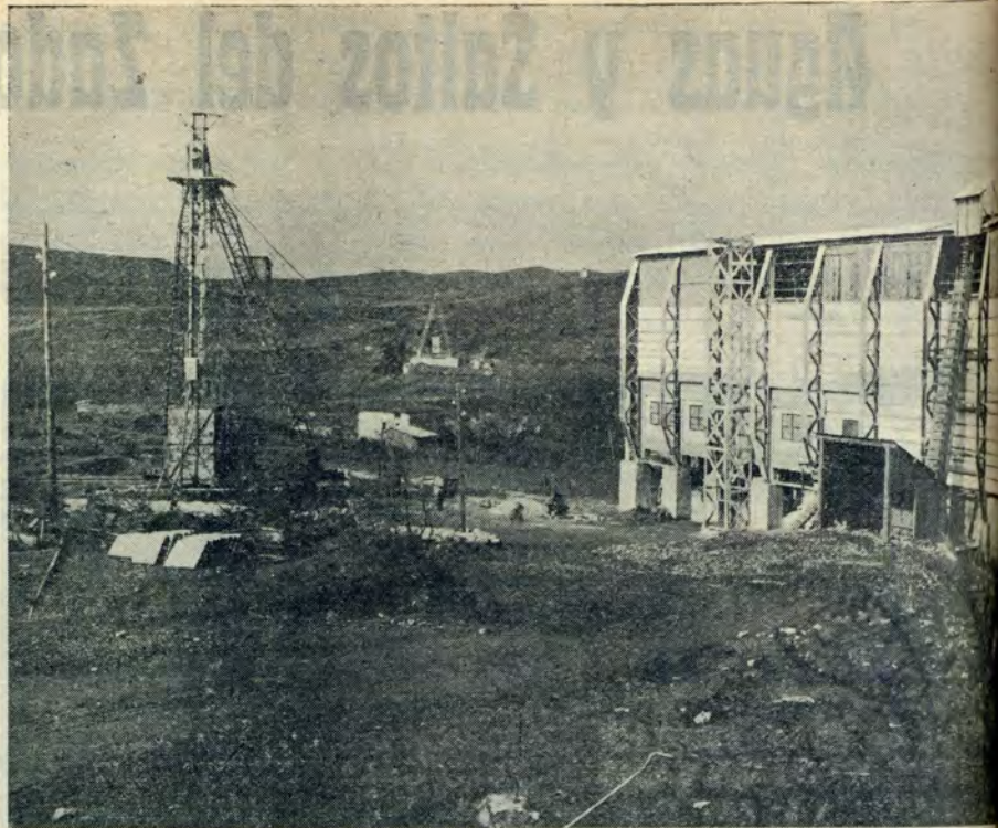
Presa de Urrúnaga.—Cable-grúa y estación de dosificación y producción de hormigón.
