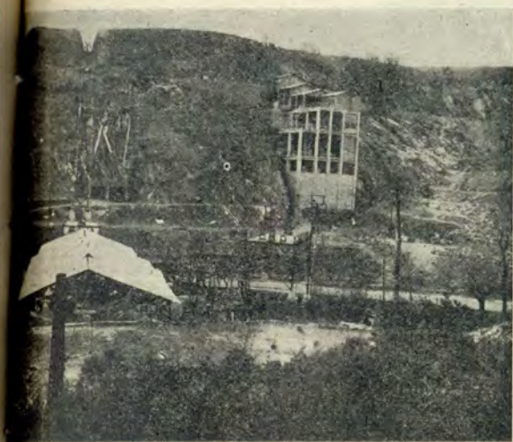
Instalación de trituración de la cantera de Landa y estación de salida del tranvía aéreo a Urrúnaga.
