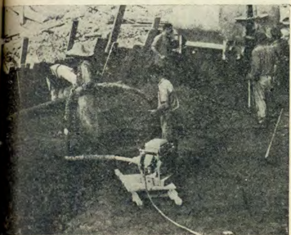
Presa de Urrunaga.—Obreros vibrando el hormigón.
