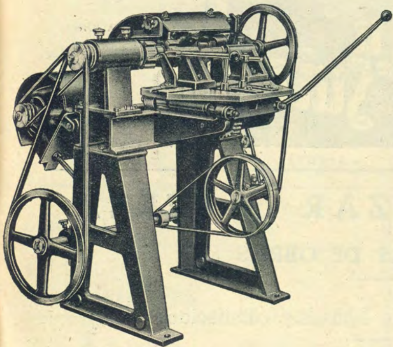
Máquina torneadora semiautomática de mangos de planchas, limas, etc., etc.
