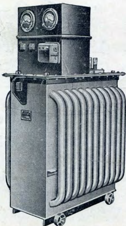
Rectificador con placas de selenio 1.500 Voltios. - 1.000 AMPS. Refrigeración por aceite
