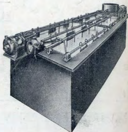
Equipo para niquelado rápido brillante, con agitación y filtración continua del electrolito. Cátodos en movimiento.
